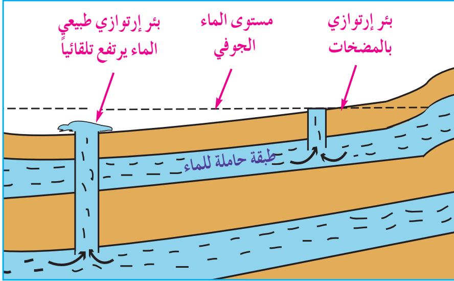
شكل (١٩) رسم توضيحي للآبار الإرتوازية
